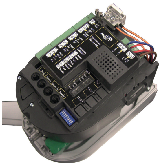
Centrale de commande pour Modus280 ou Modus420
