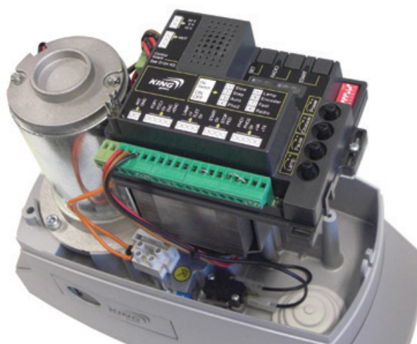
Centrale de commande pour Dynamos 24
