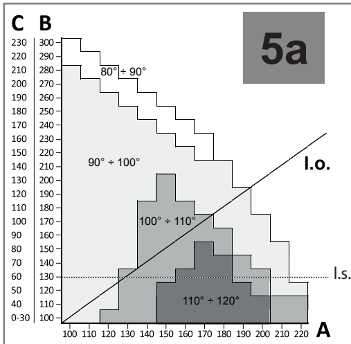
Fig. 5 IT - Grafico angolo di apertura EN - Opening angle graph DE - Zeichnung zum Öffnungswinkel ES - Gráfico ángulo de apertura
